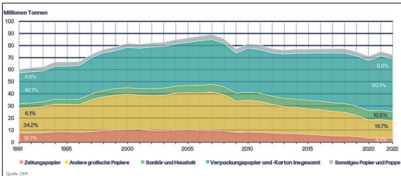
VERBRAUCH VON PAPIER UND PAPPE NACH SORTEN IN EUROPA
